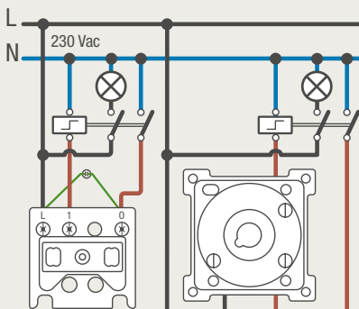
170-70015 170-70001 DRUKKNOP NORMAAL OPEN CONTROLÉ
