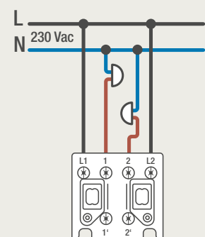
170-75015 / 170-75001 DUBBELE DRUKKNOP 2 x NORMAAL OPEN
