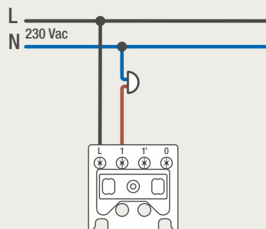
170-73015 / 170-73001 DRUKKNOP NORMAAL OPEN OF NORMAAL GESLOTEN
